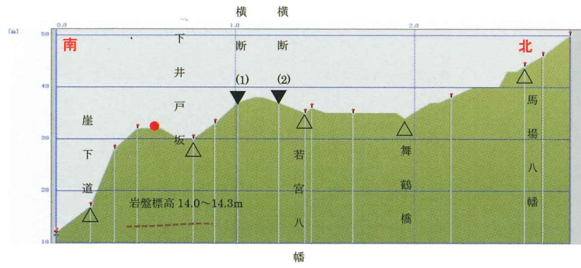
図-9 常陸太田市街地の縦断面図
