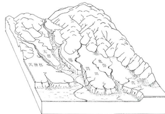
図-5 下末吉海進後海面低下時代の地形想定図 (出典：1)
